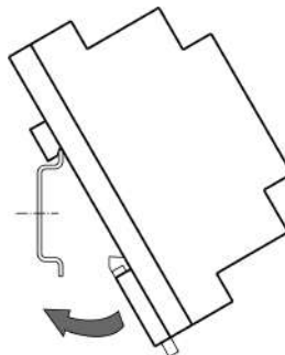
Рисунок 4.9 – Монтаж прибора с креплением на DIN-рееку
